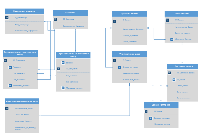
Рисунок 15 - «ER-модель» предметной области управления взаиморасчетами с клиентами компании ООО «Тат Телеком»
