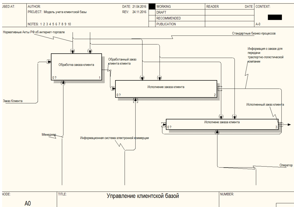
Рисунок 5 - Диаграмма декомпозиции А0.
