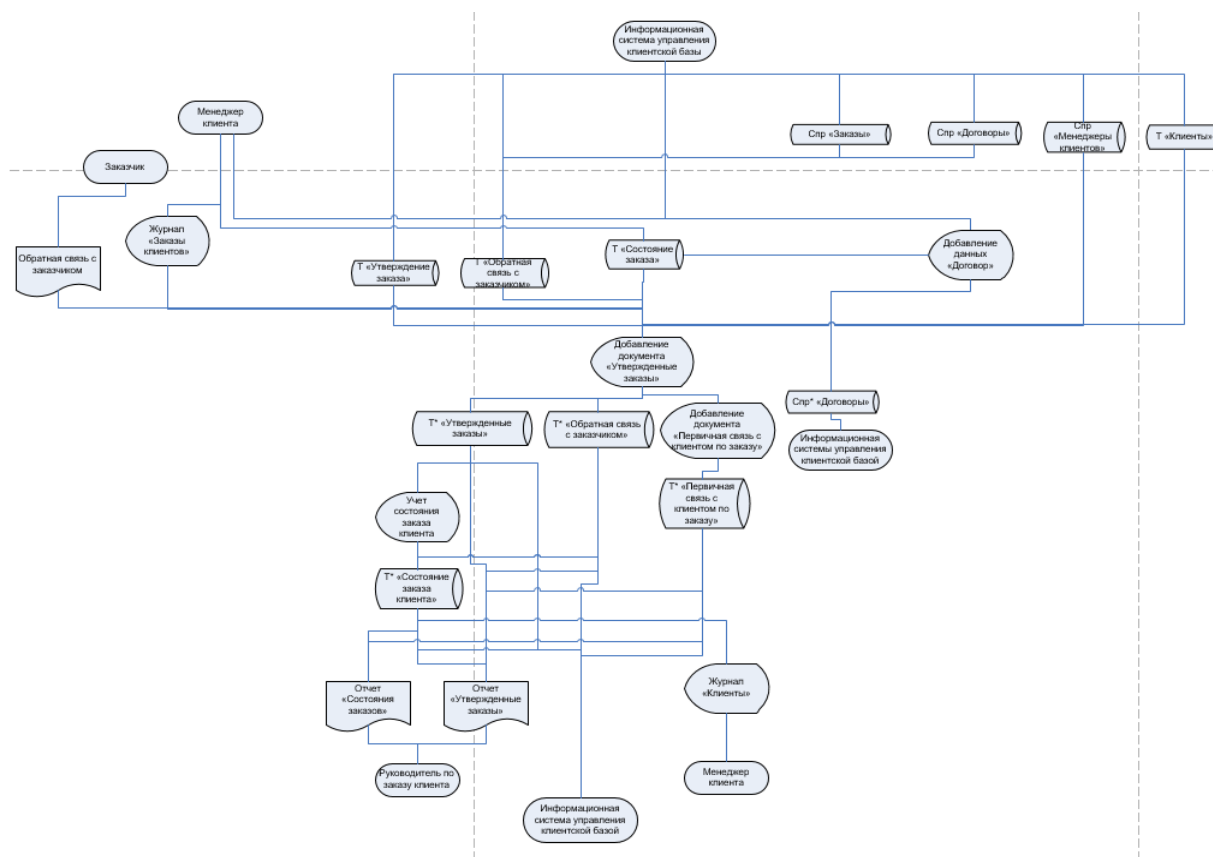
Рисунок 12 - Информационная модель системы автоматизации взаиморасчетами с клиентами
